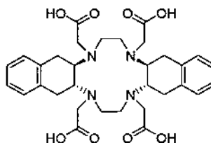
trans-syn-trans
